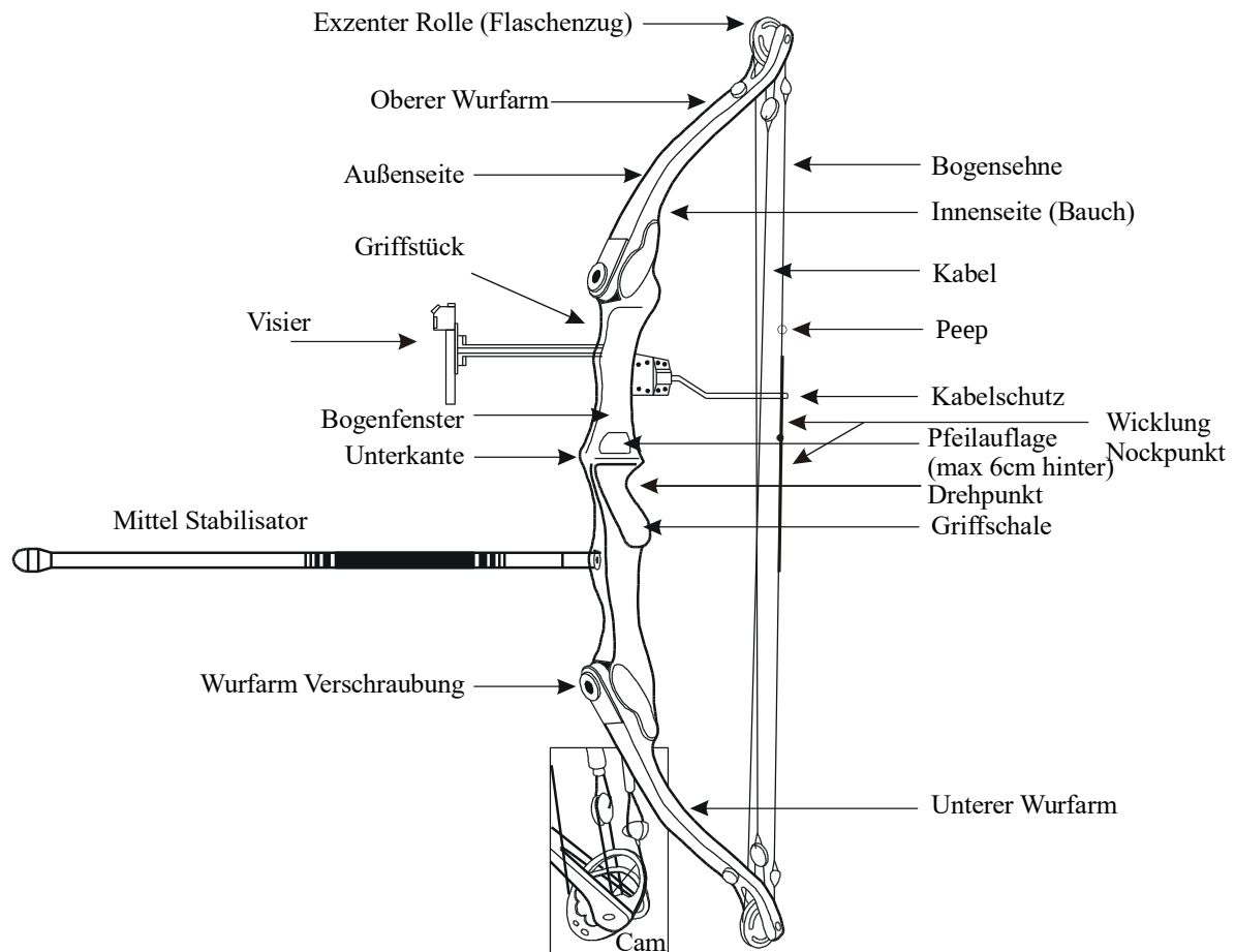
Abbildung 17: Beschreibung des Compound-Bogens
